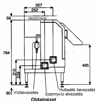
Oldalnézet
