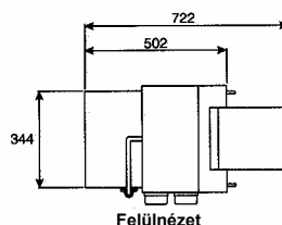
Felülnézet
